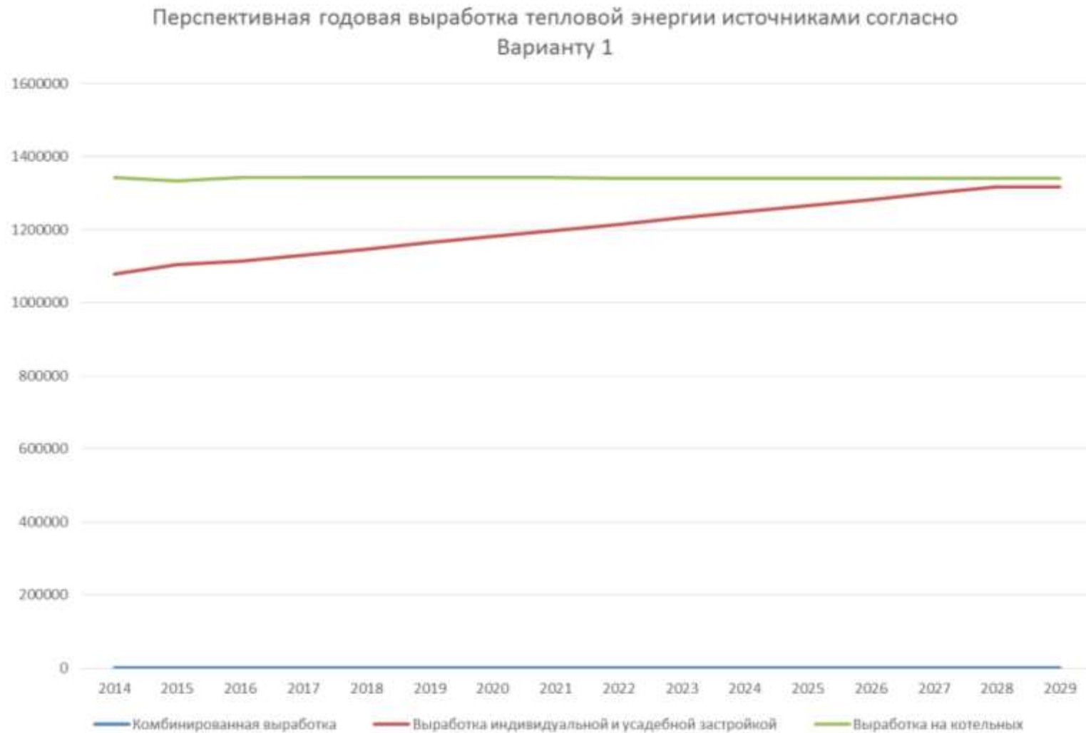
Рисунок 2.1 – Перспективная годовая выработка тепловой энергии источниками согласно Варианту 1 (Гкал/год)
