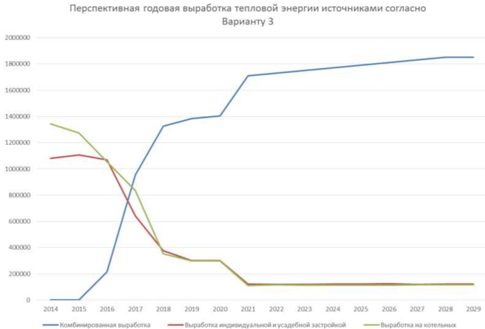
Рисунок 4.1 – Перспективная годовая выработка тепловой энергии источниками согласно Варианту 3
