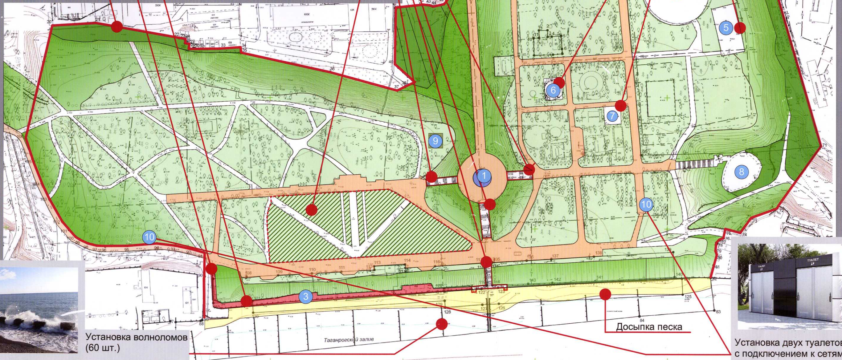
Устройство металлического ограждения территории h=2.2 м.
