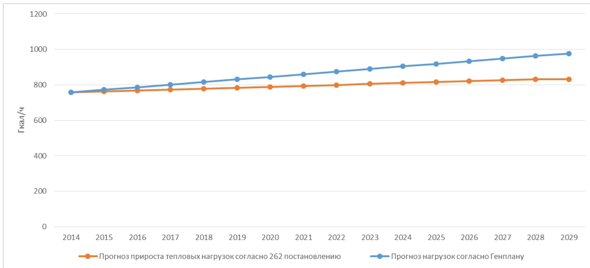
Рисунок 4 - Динамика прироста тепловой нагрузки согласно Генплану и 262 постановлению Прирост тепловой нагрузки, рассчитанный согласно 262 постановлению, на 25% ниже, чем нагрузка, приведённая в Генплане.
