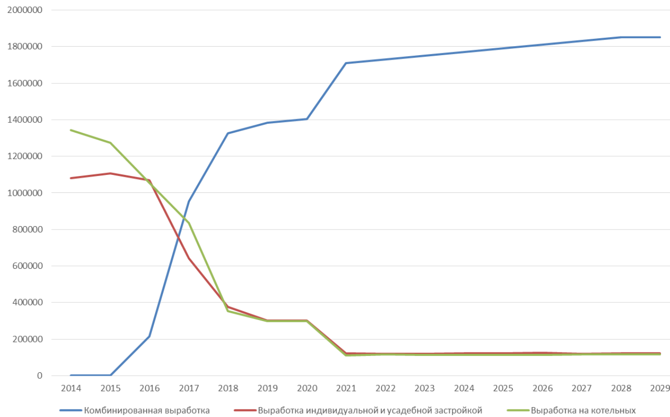
Рисунок 12 - Перспективная годовая выработка тепловой энергии источниками согласно Варианту 3 (Гкал/год)
