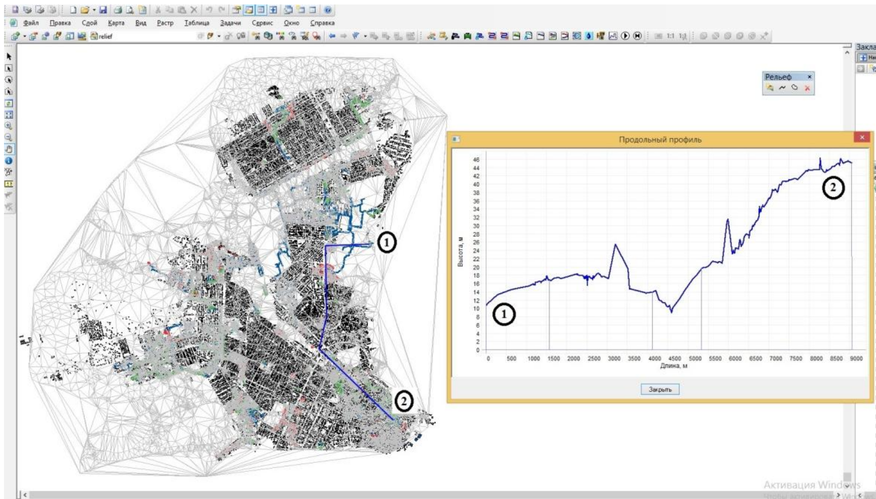
Рисунок 5.2б– Продольный профиль трассы от места расположения ПГУ ТЭЦ 2 (1) до потребителя (2)
