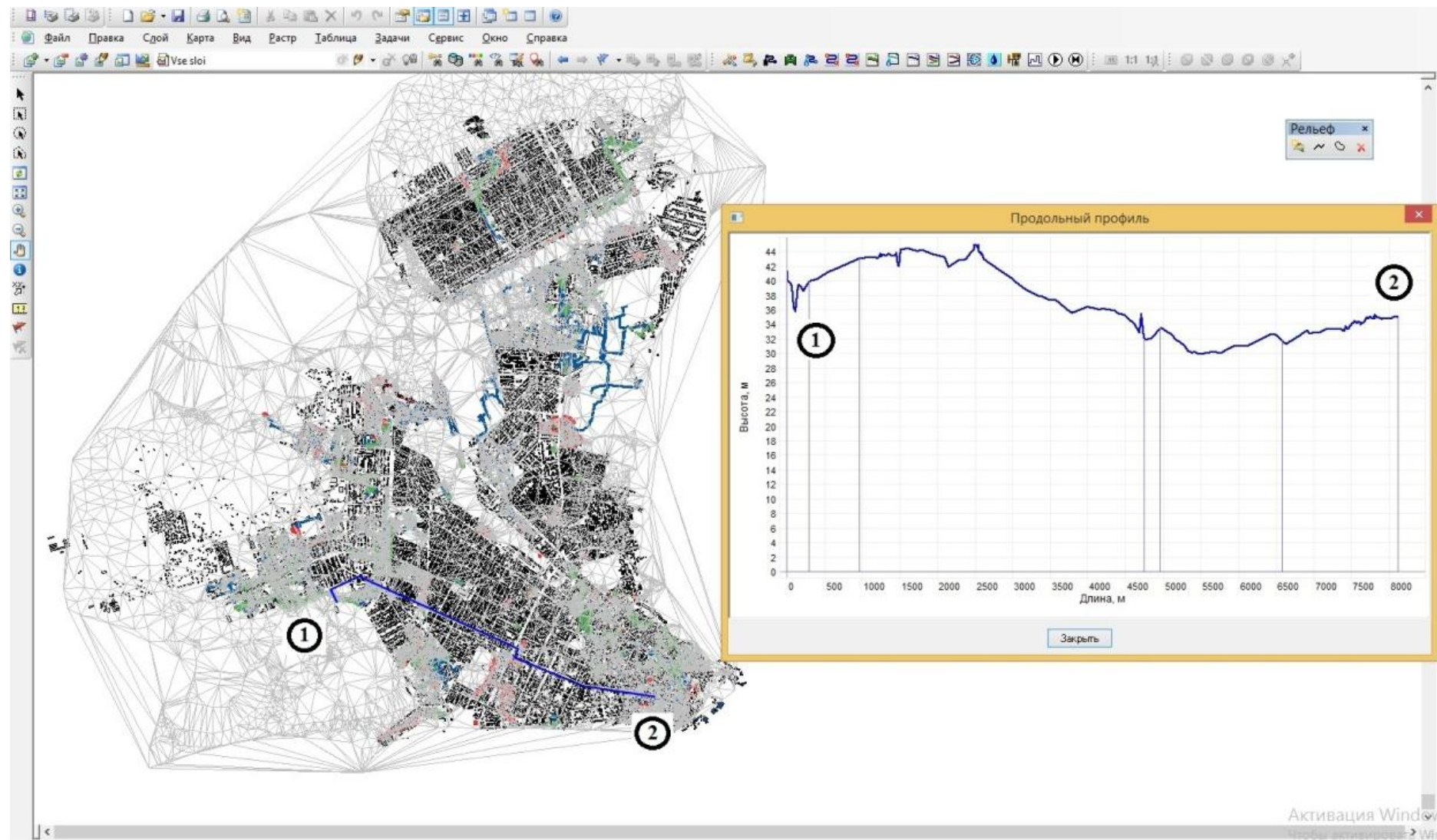
Рисунок 5.2а – Продольный профиль трассы от места расположения ПГУ ТЭЦЗ (1) до потребителя (2)
