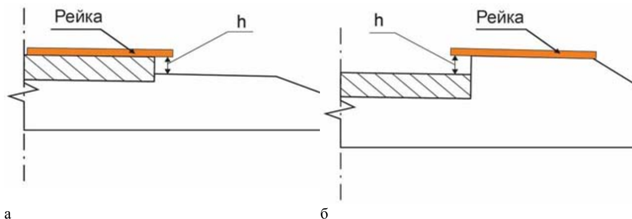
Рисунок 1 - Схема измерения величины занижения (возвышение) обочины и разделительной полосы: а - при занижении; б - при возвышении
